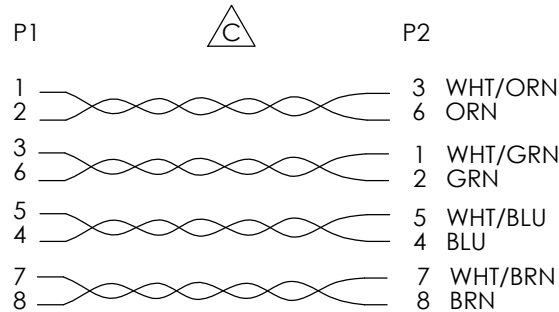
WIRING MAP
