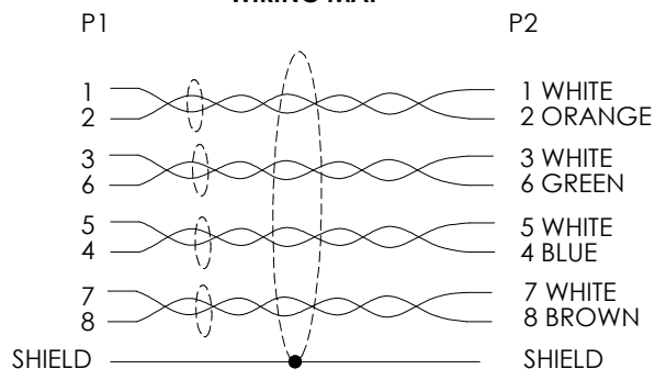
WIRING MAP
