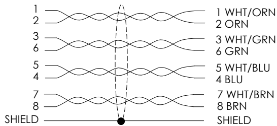
P1 WIRING MAP P2
