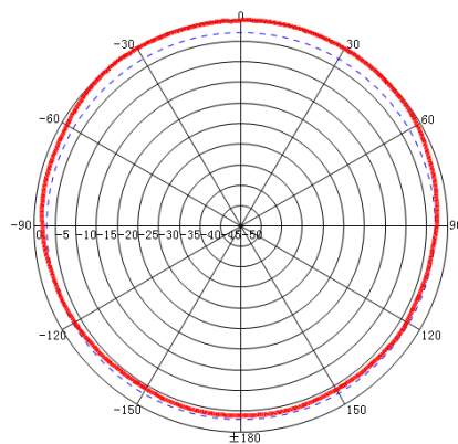
H-Plane: 2500 MHz
