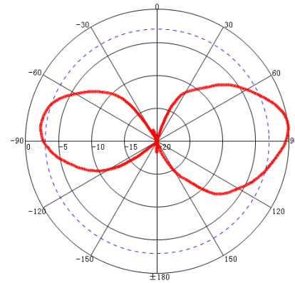
V-Plane: 2400 MHz
