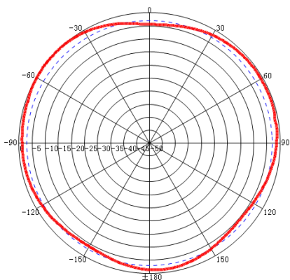
H-Plane: 5500 MHz
