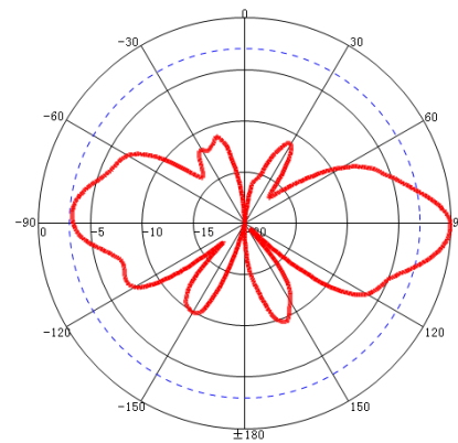
V-Plane: 2400 MHz
