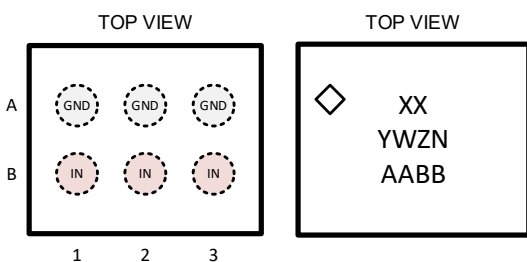
WLCSP32-6
