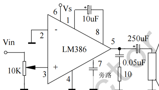
图 2 放大器增益=200
