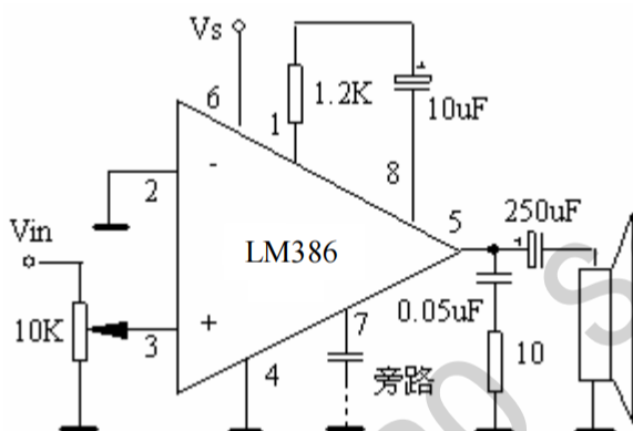
图 3 放大器增益=50
