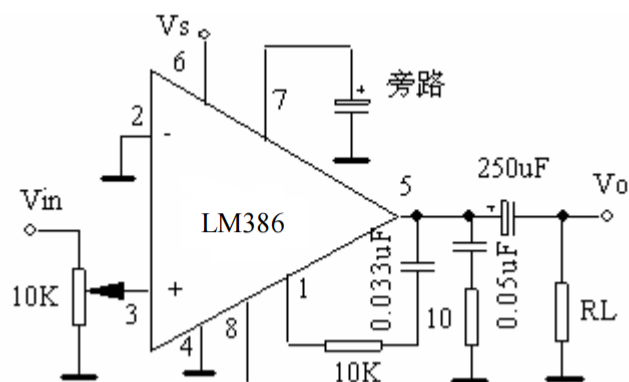
图 5 低频提升放大器
