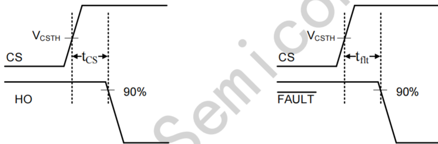
图 6-4 CS关断时间定义
