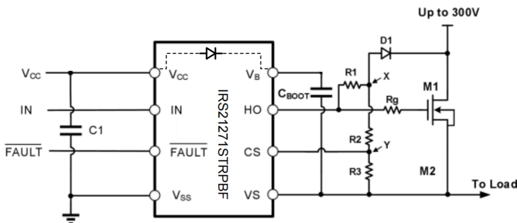
图 7-2 典型应用电路图
