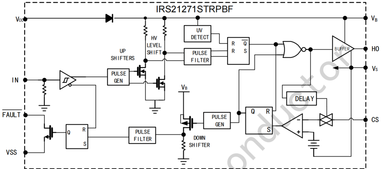
图 7-1 功能框图
