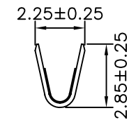
SEC:B-B
