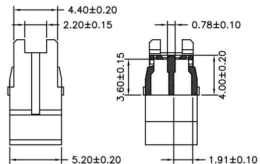
SEC:A-A
