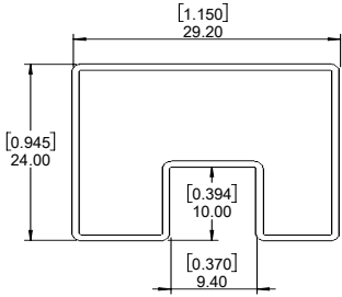
包装管尺寸图
