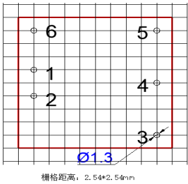
推荐 PCB 图
