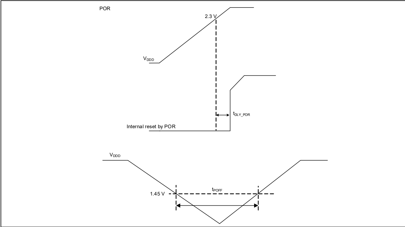
Figure 26-15 POR specifications
