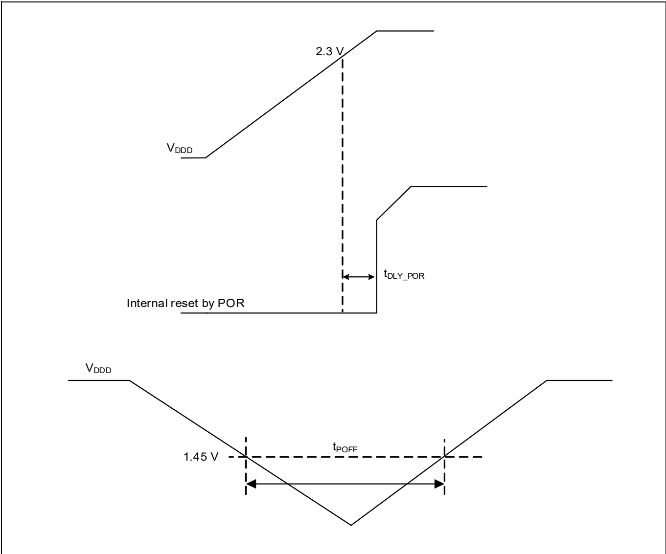
Figure 25 POR specifications
