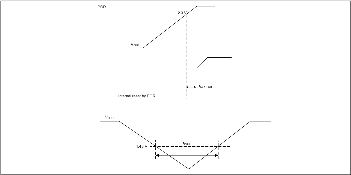
Figure 24 POR specifications
