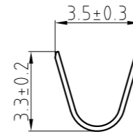
剖面 A-A
