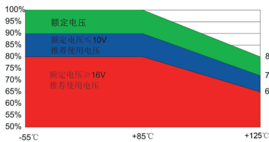
图5. 高分子型产品工作电压
