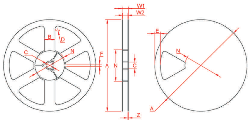
图3 轮盘尺寸图
