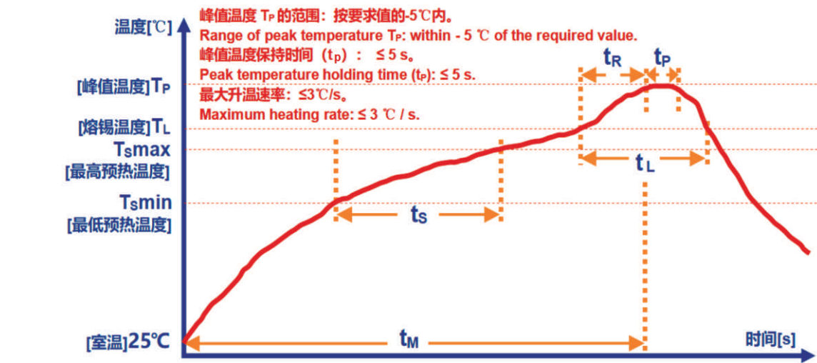
图7. 回流焊温度时间曲线图
