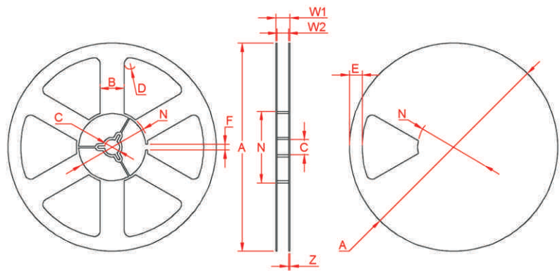
图3 轮盘尺寸图
