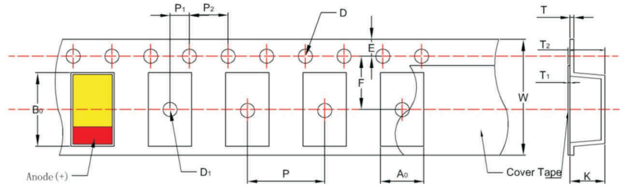
图2载带尺寸图
