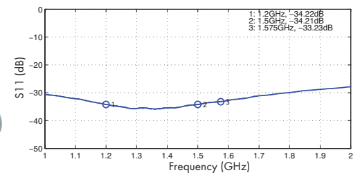
S-parameters
