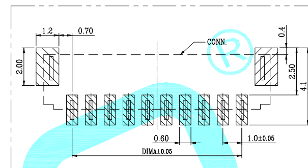
P.C.B LAYOUT
