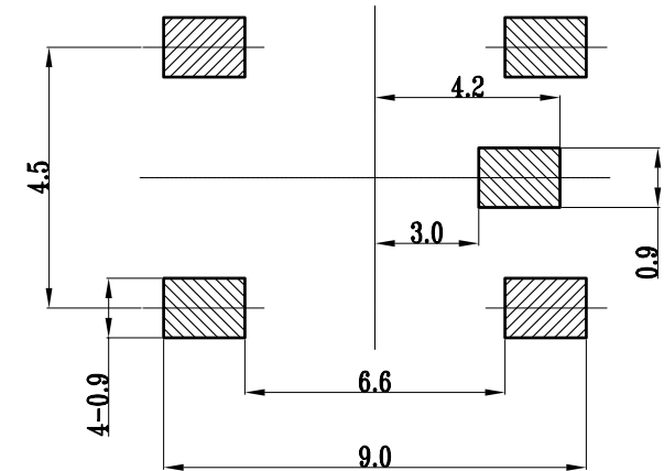
P.C.B LAND DIMENSION
