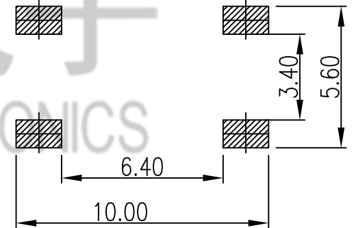
PCB. 焊接图
