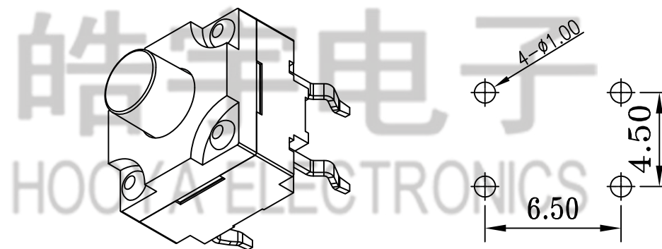
PCB. 焊接图
