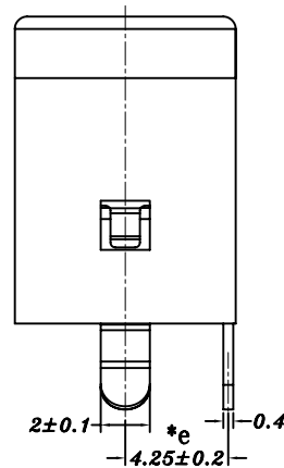
VIEW A-A
