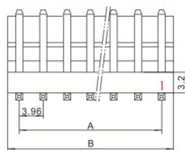
HX39603-WAG (5274/3.96)
