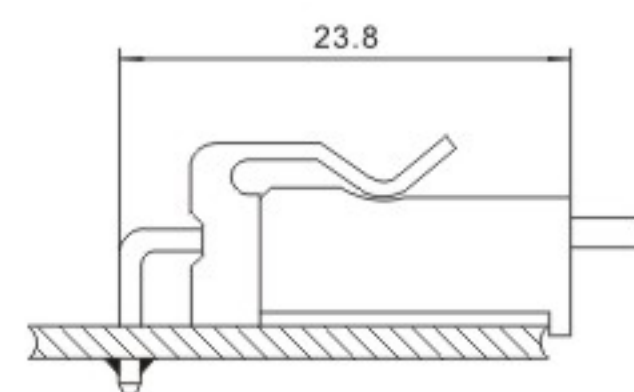
针座 WAFER (5273/5274/5271/3.96)
