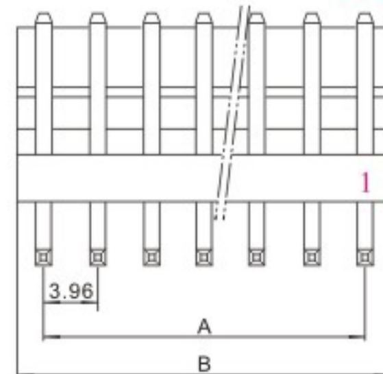
HX39603-WAG (5274/3.96)
