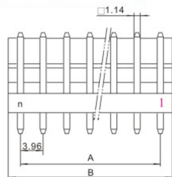
HX39603-A (5273/3.96)
