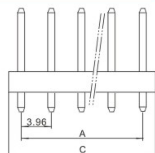
HX39603-A (5273/3.96)
