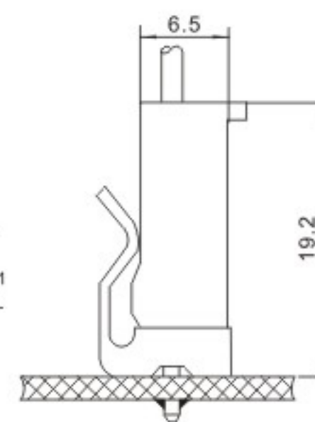
针座 WAFER (5273/5274/5271/3.96)
