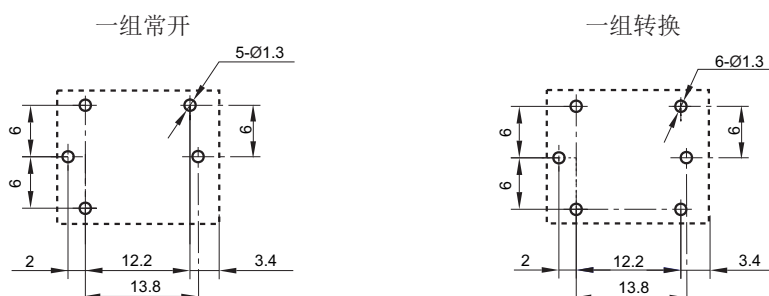
安装孔尺寸(底视图)
