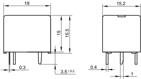
外形图
