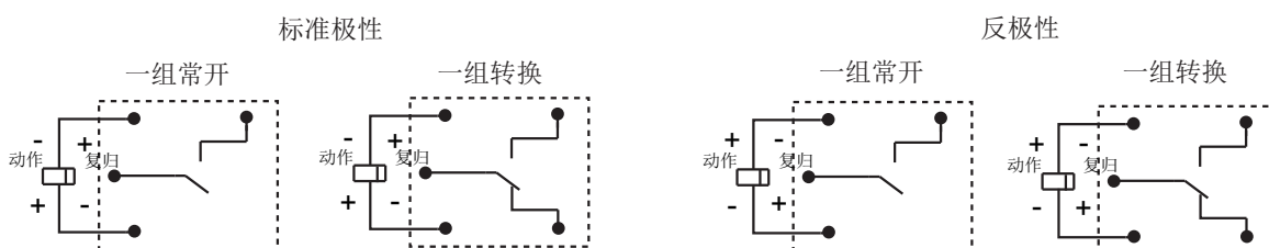
接线图(底视图)
