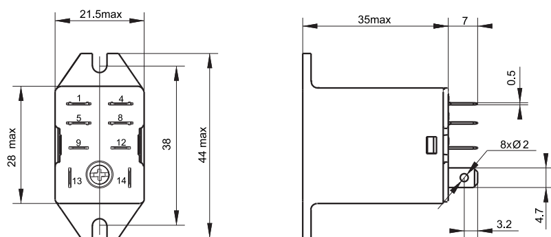
外形图
