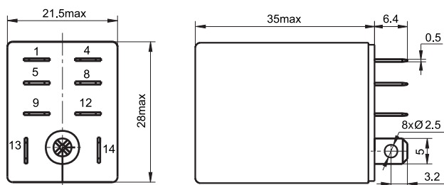
外形图
