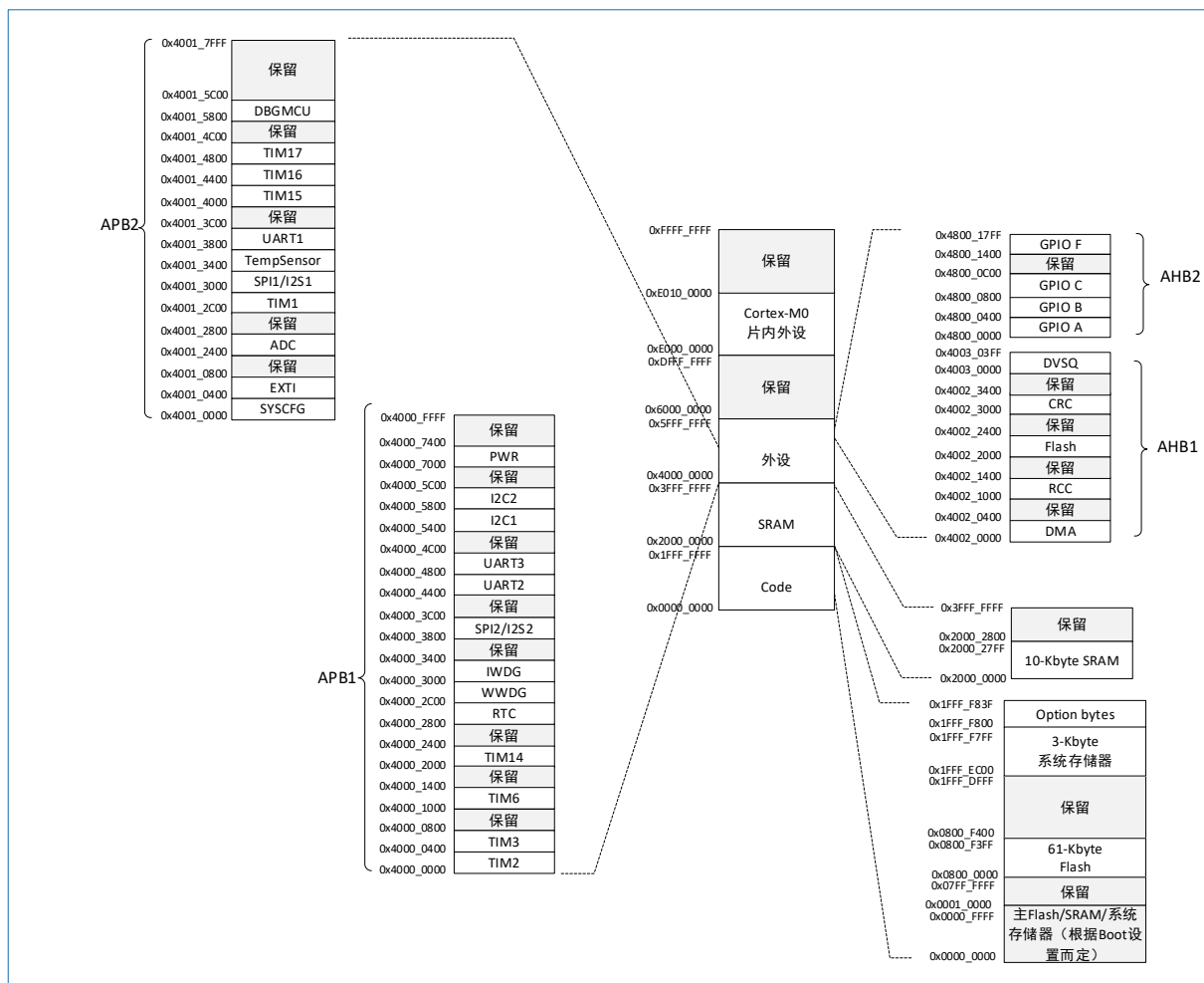
图 3-2 HK32R78x 存储器映射
