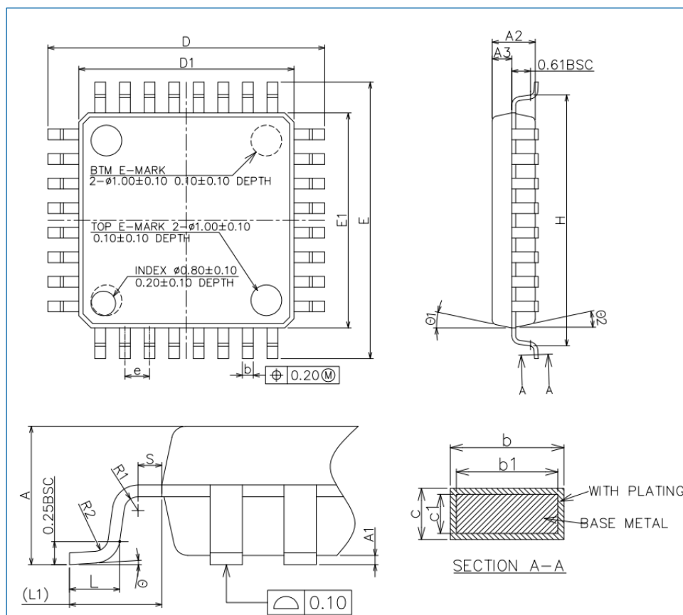
图 7-2 LQFP32 封装尺寸
