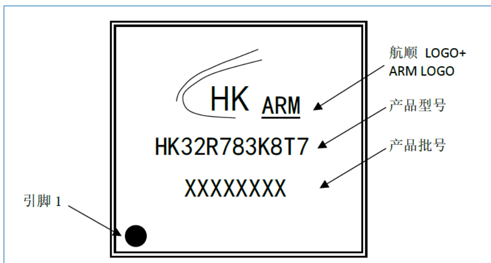
图 7-6 LQFP32 丝印示例
