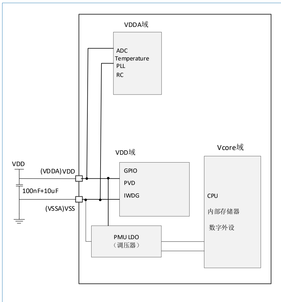
图 5-1 电源框图
