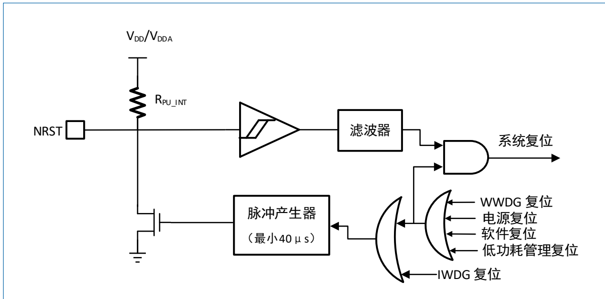
图 3-3 复位信号
