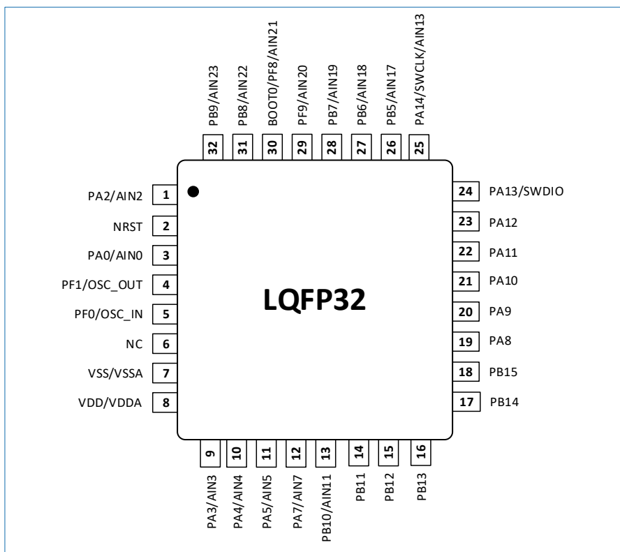
图 6-2 LQFP32 封装引脚排列
