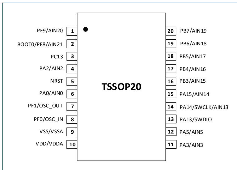
图 6-4 TSSOP20 封装引脚排列
