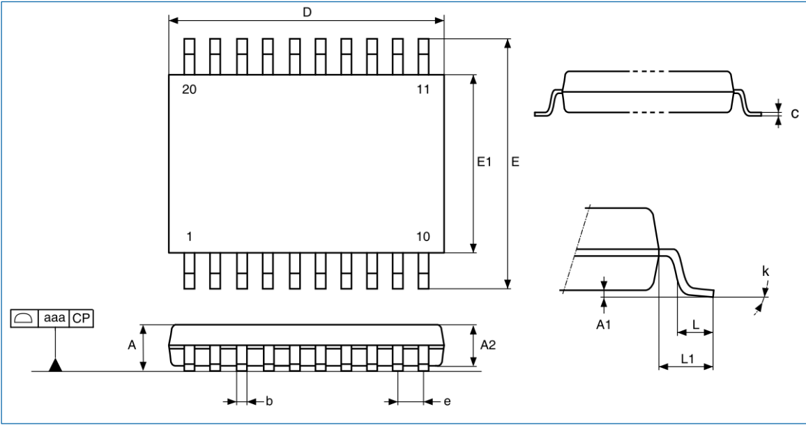
图 7-4 TSSOP20 封装尺寸
