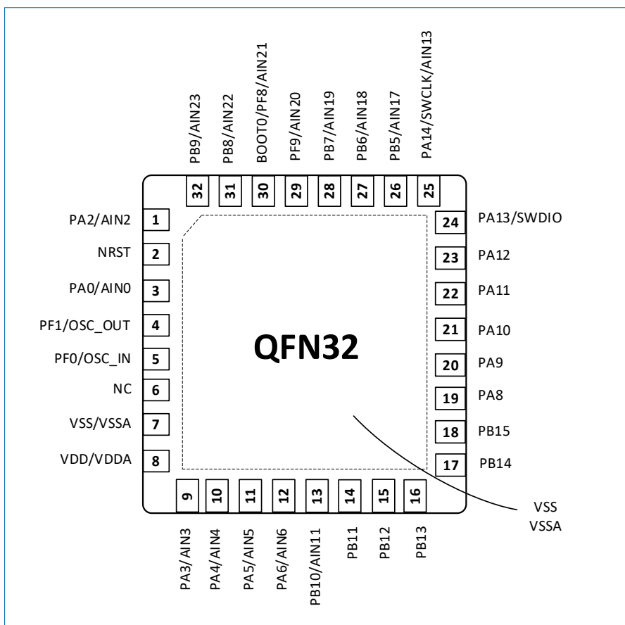
图 6-3 QFN32 封装引脚排列
