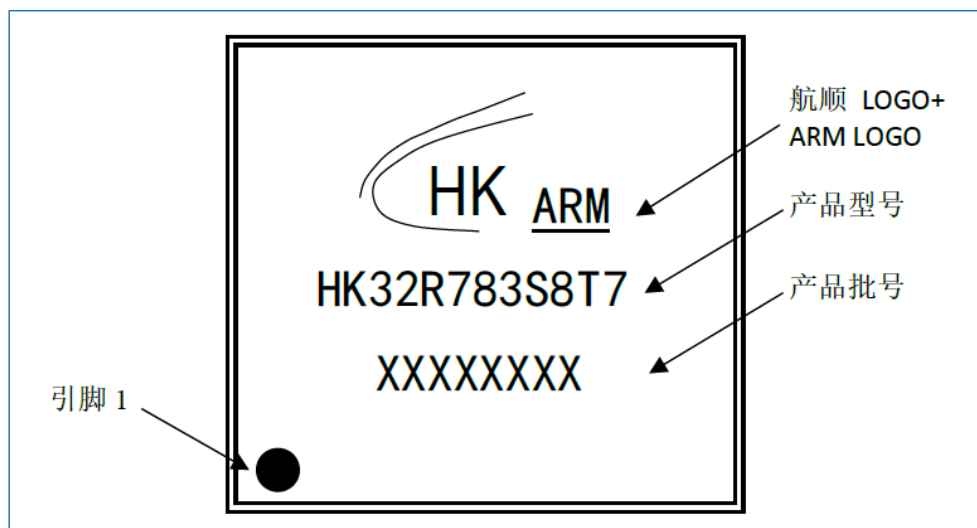
图 7-5 LQFP44 丝印示例
