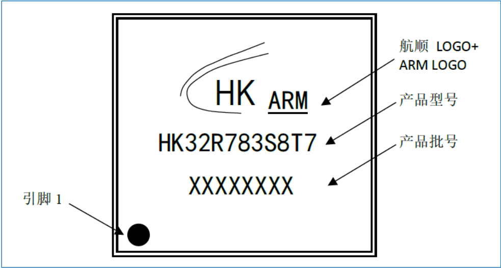
图 7-5 LQFP44 丝印示例
