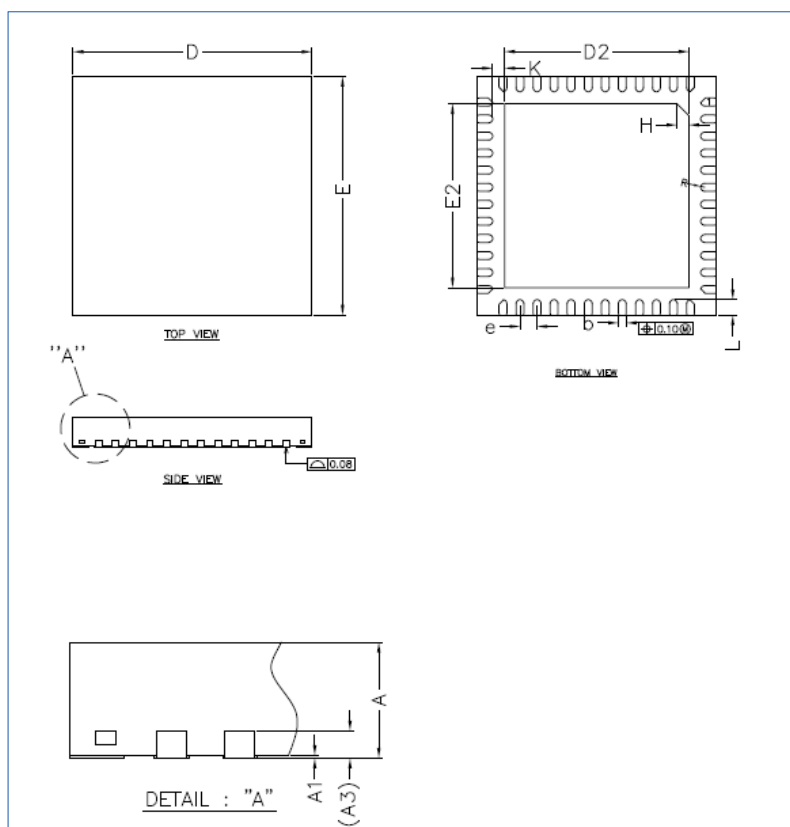
图 7-3 QFN48 封装尺寸
