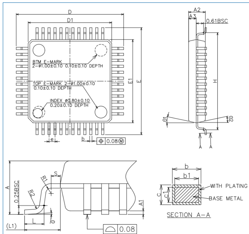
图 7-4 LQFP48 封装尺寸
