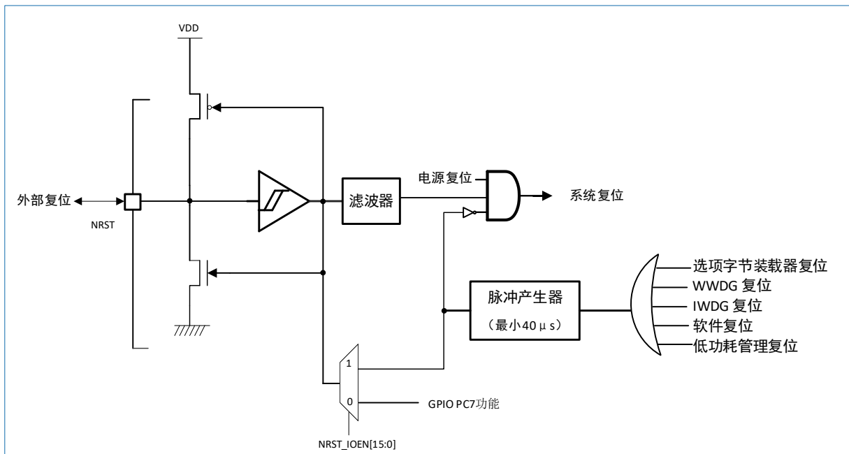
图 3-3 复位信号
