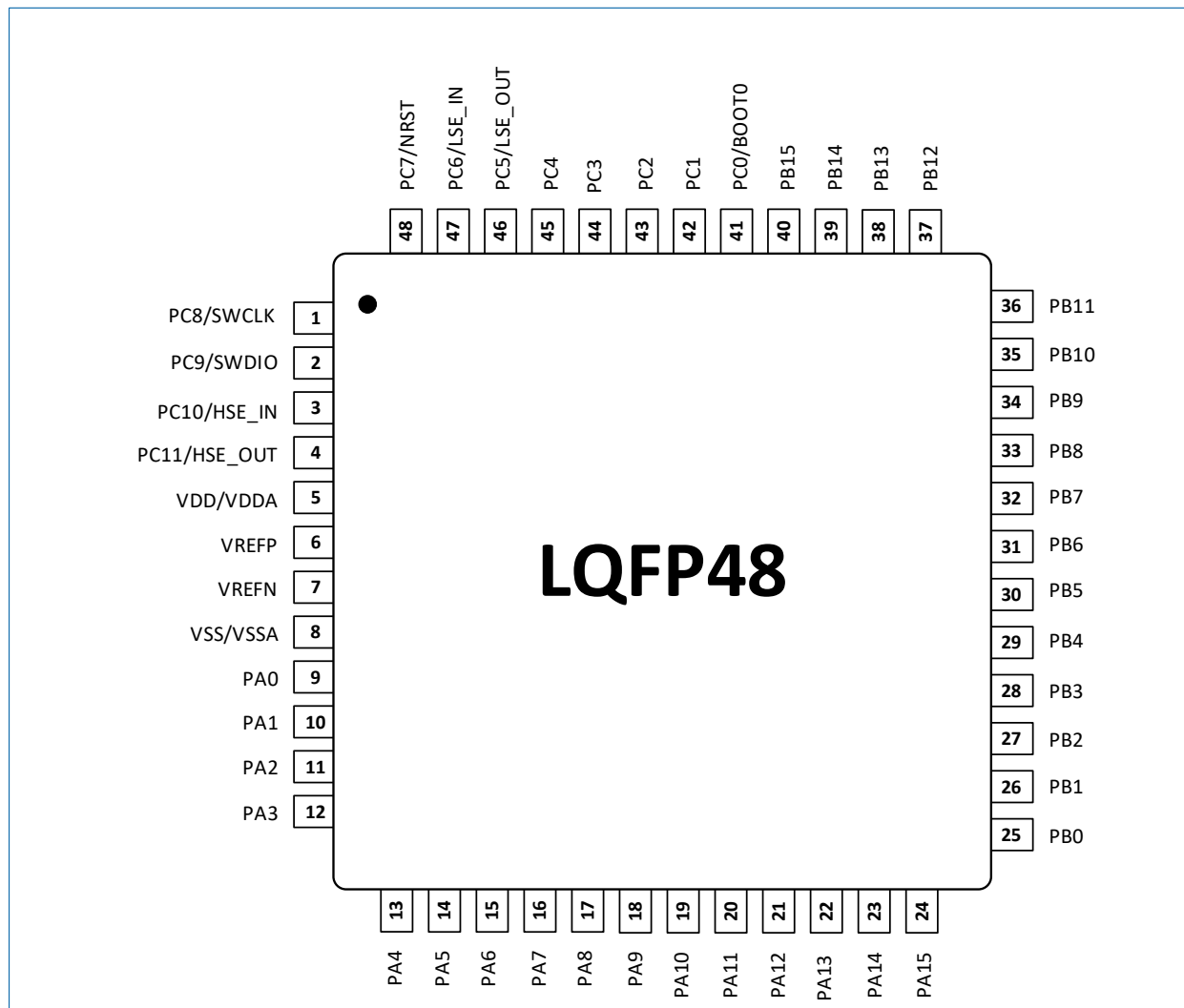
图 6-4 LQFP48 封装引脚排列
