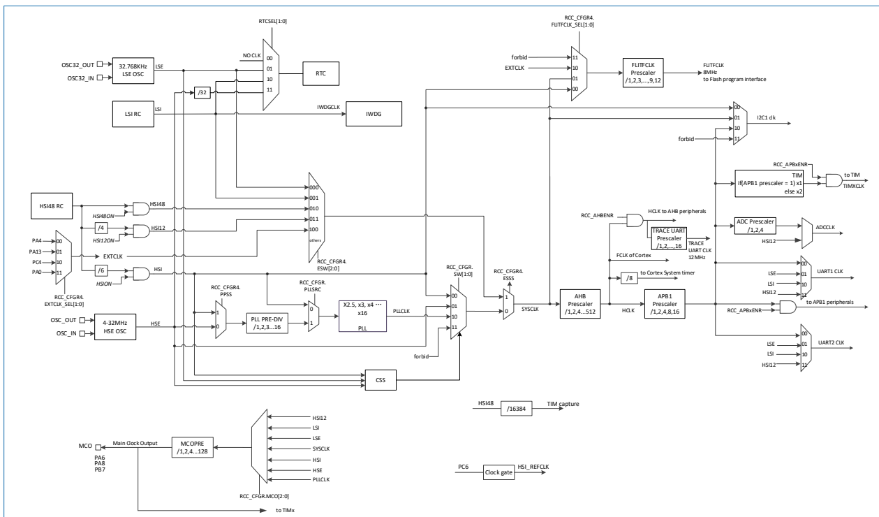
图 3-4 时钟树
