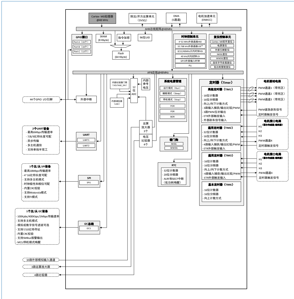
图 3-1 HK32M060C8T7 功能框图
