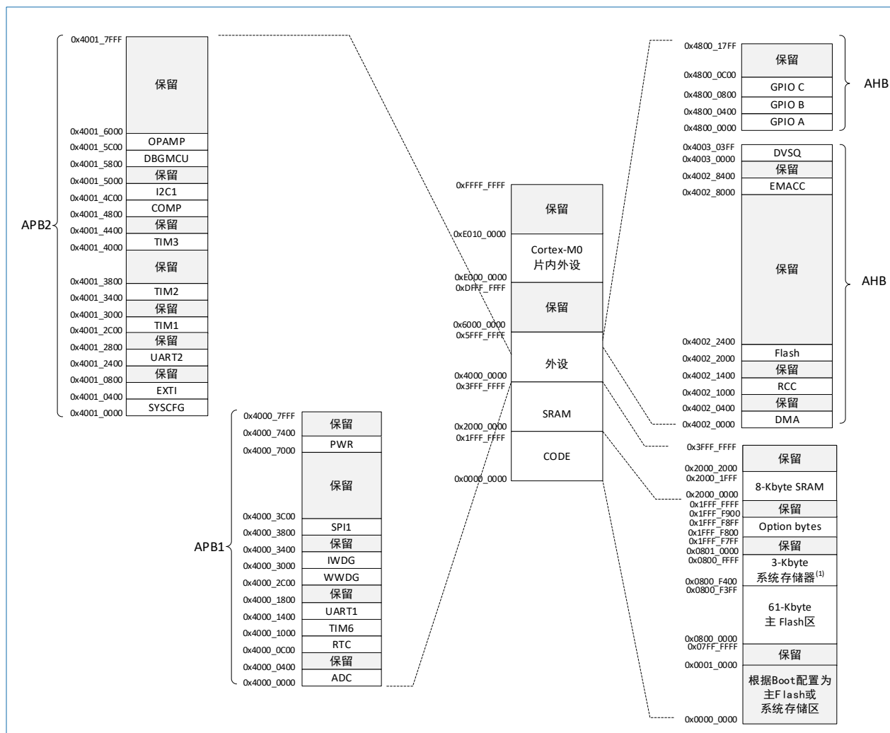
图 3-2 HK32M060C8T7 存储器映射
