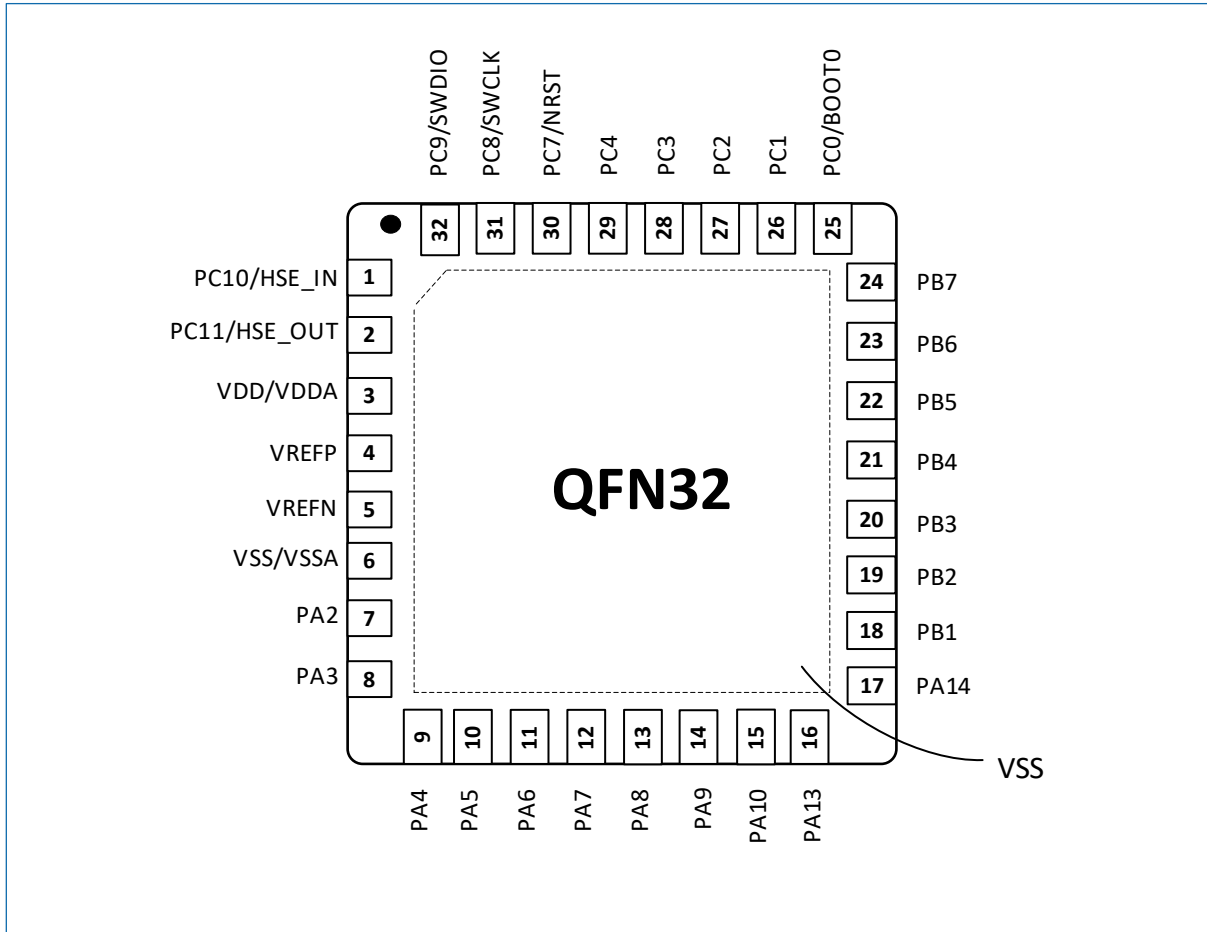
图 6-1 QFN32 封装引脚排列
