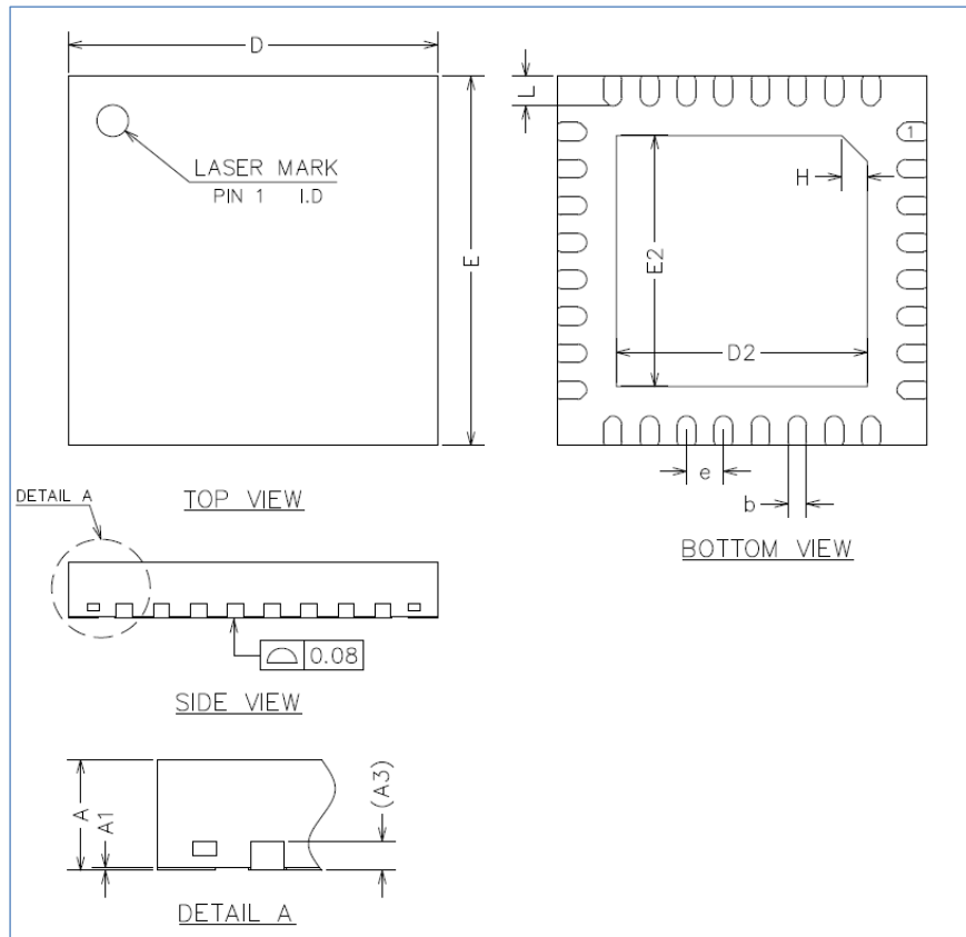
图 7-1 QFN32 封装尺寸
