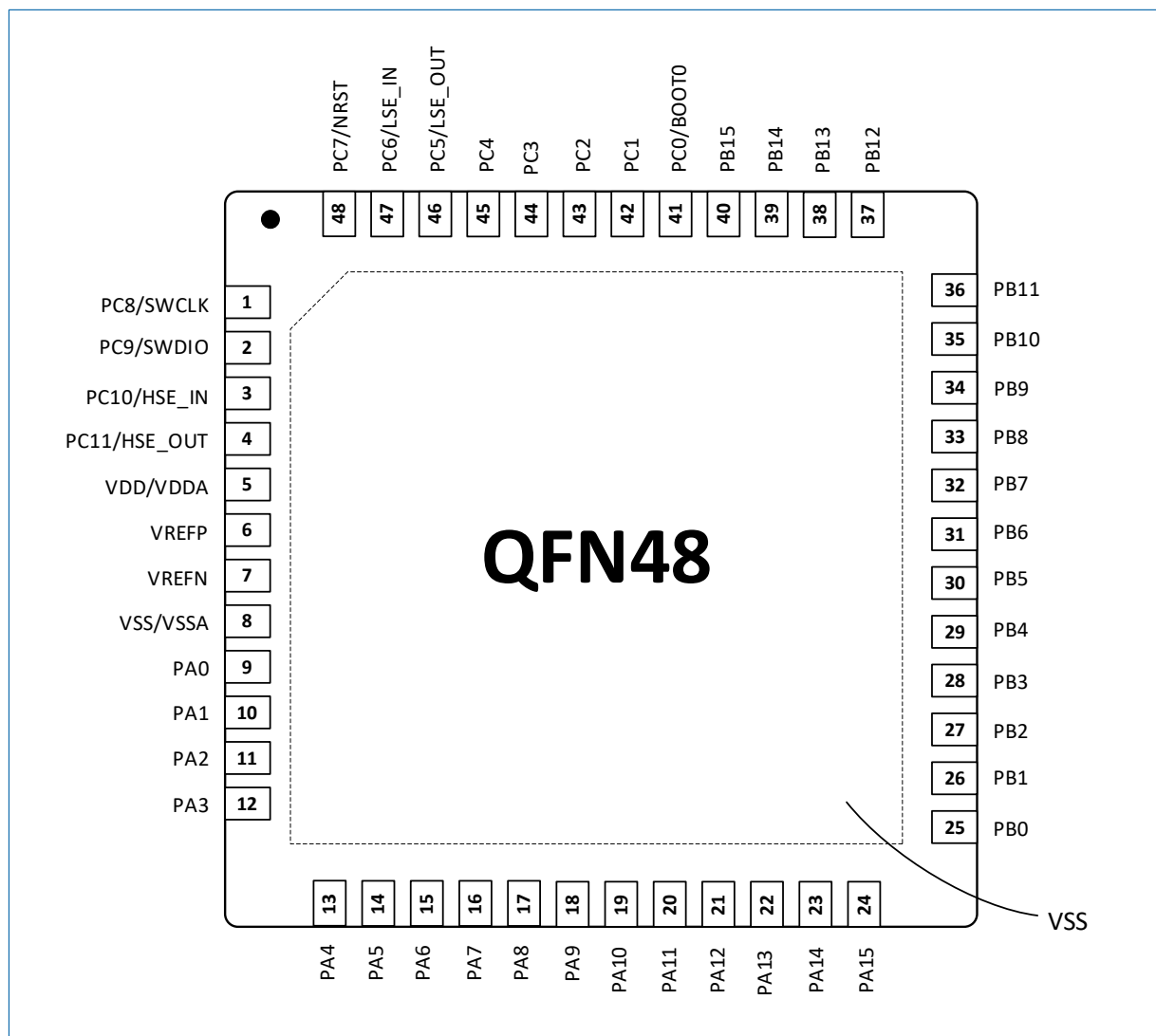
图 6-3 QFN48 封装引脚排列
