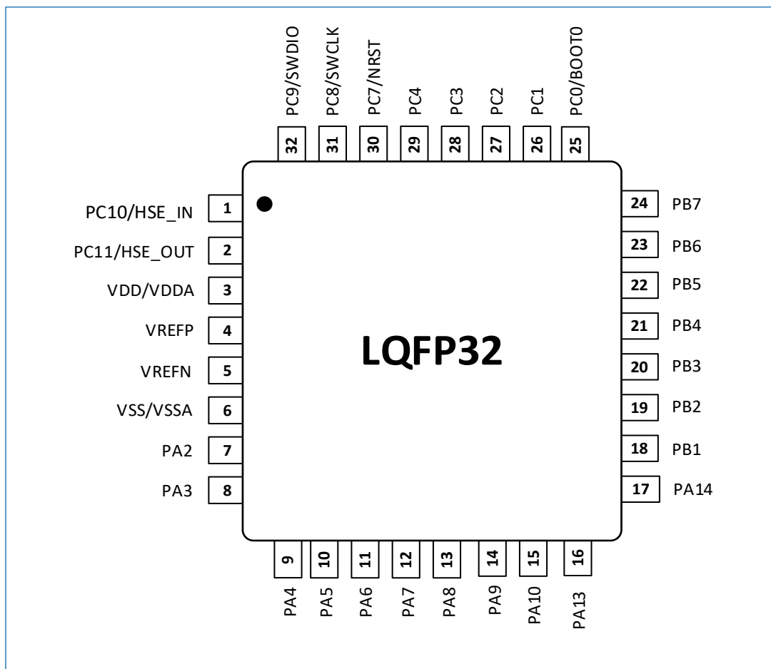
图 6-2 LQFP32 封装引脚排列
