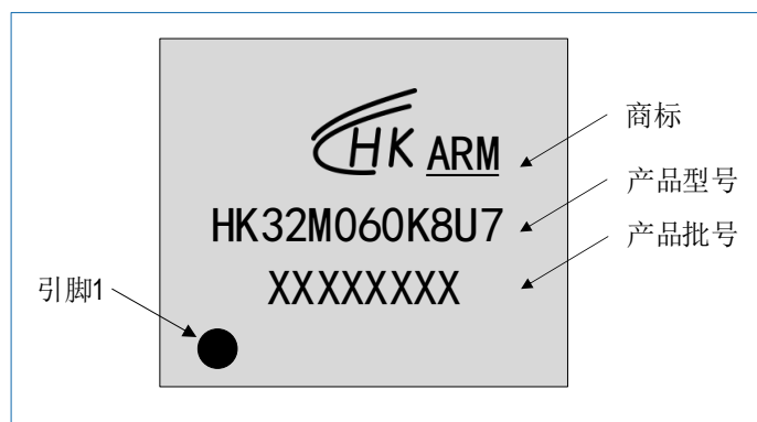
图 7-5 QFN32 HK32M060K8U7 丝印示例
