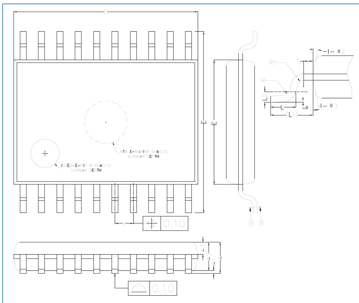
图 7-5 TSSOP20 封装尺寸
