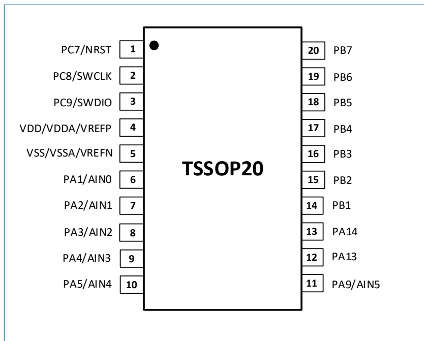
图 6-5 TSSOP20 封装引脚排列
