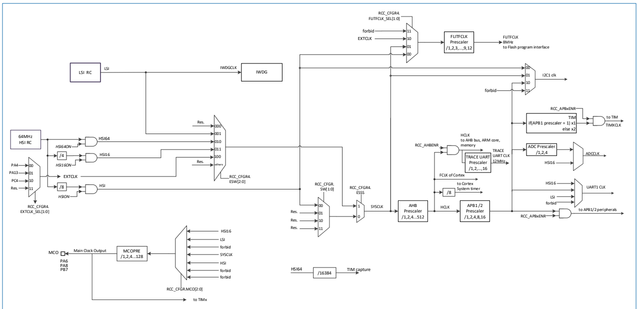
图 3-4 时钟树
