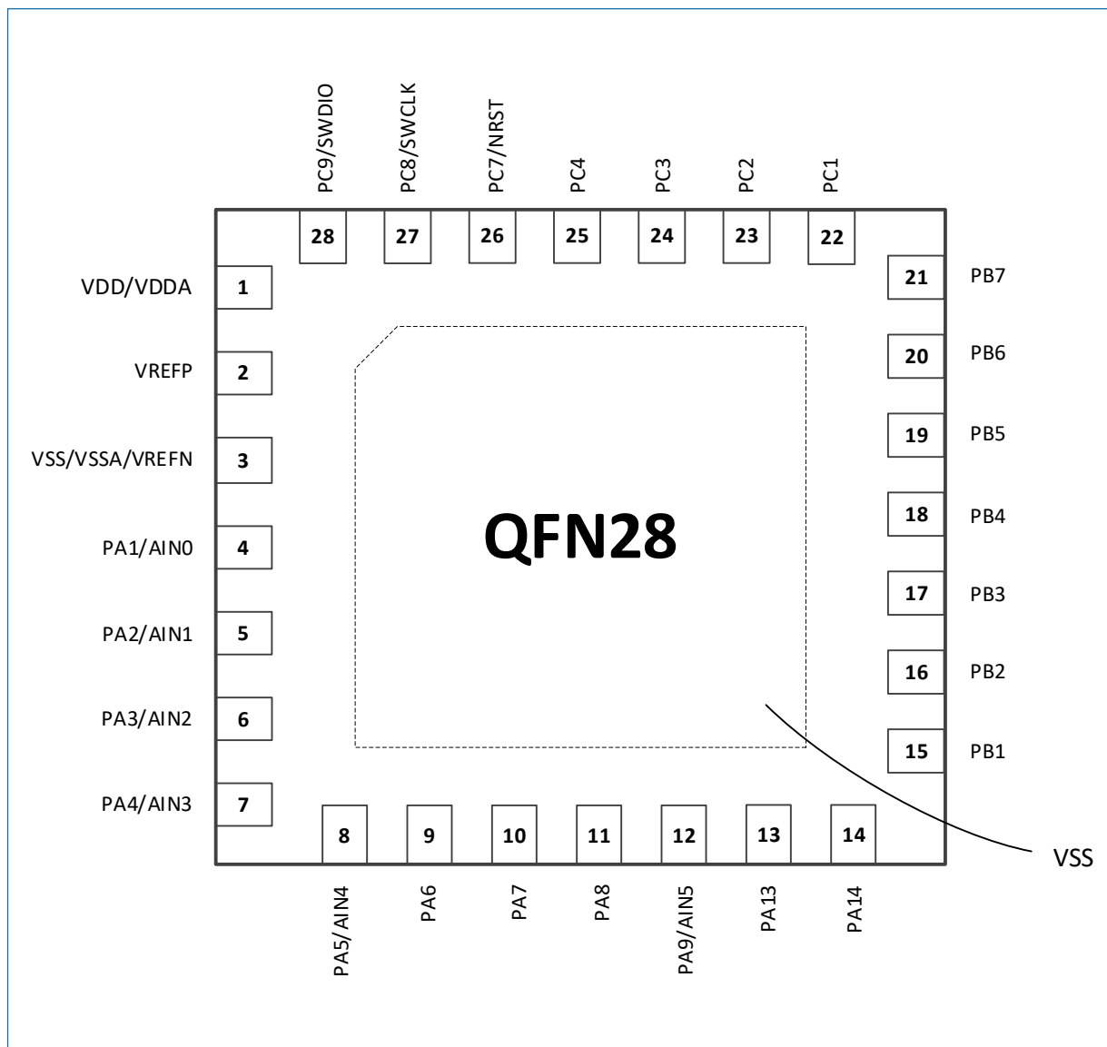
图 6-2 QFN28 封装引脚排列
