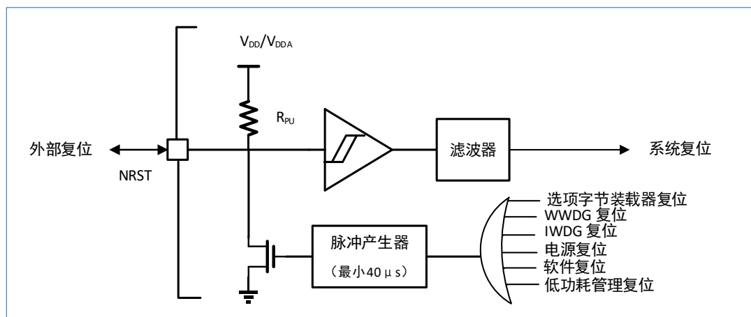
图 3-3 复位信号
