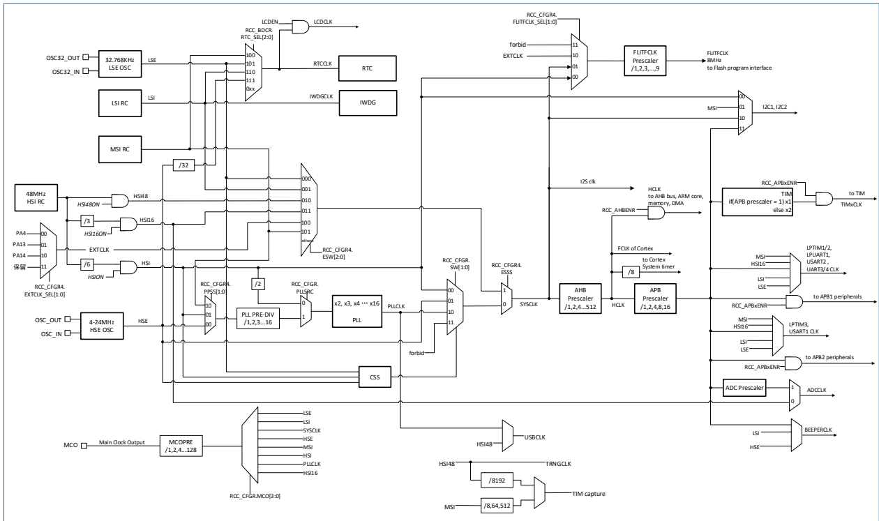
图 3-4 时钟树
