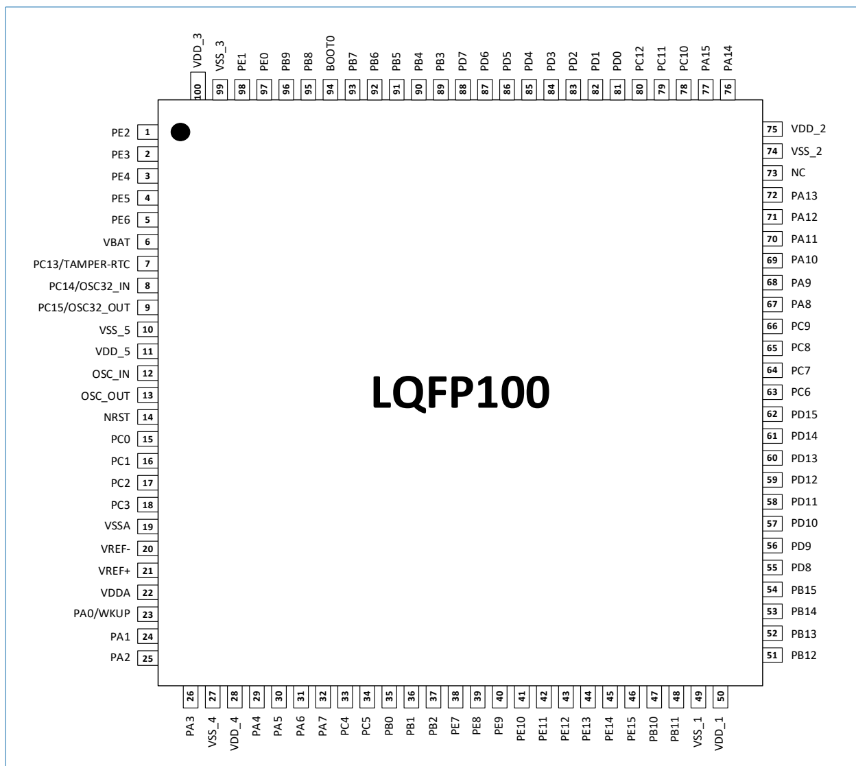
图 6-2 LQFP100 封装
