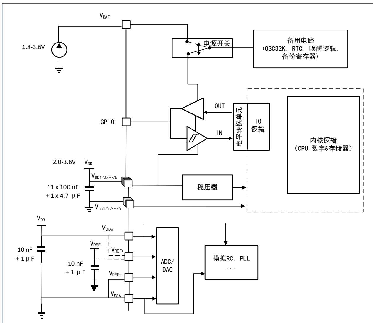
图 5-1 电源供电
