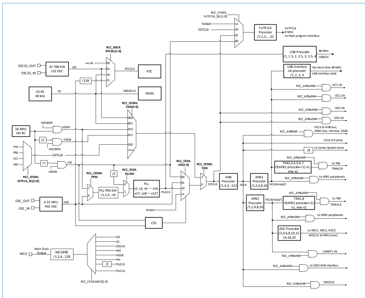
图 3-4 时钟树
