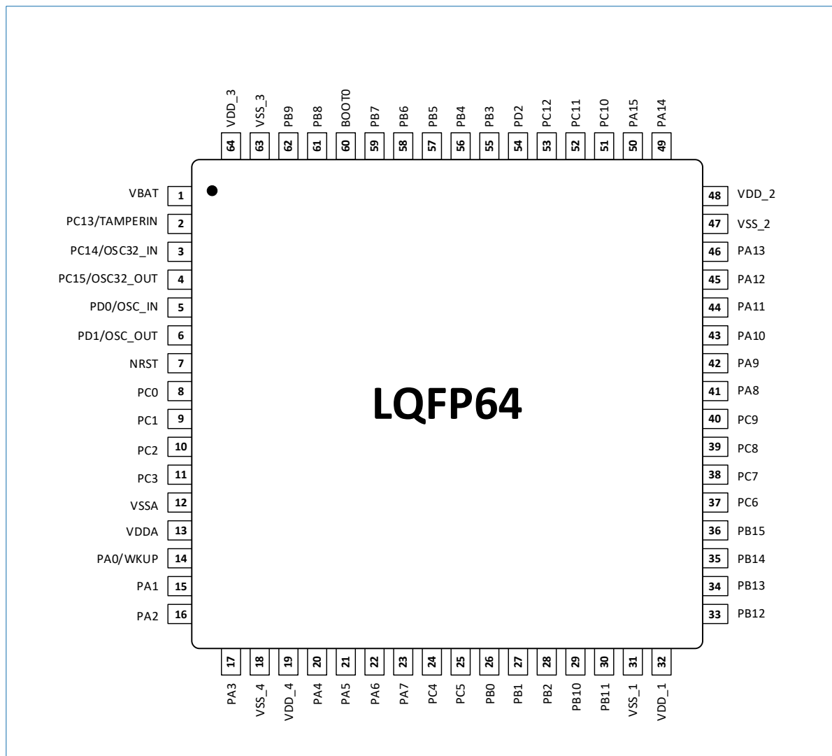
图 5-3 LQFP64 封装
