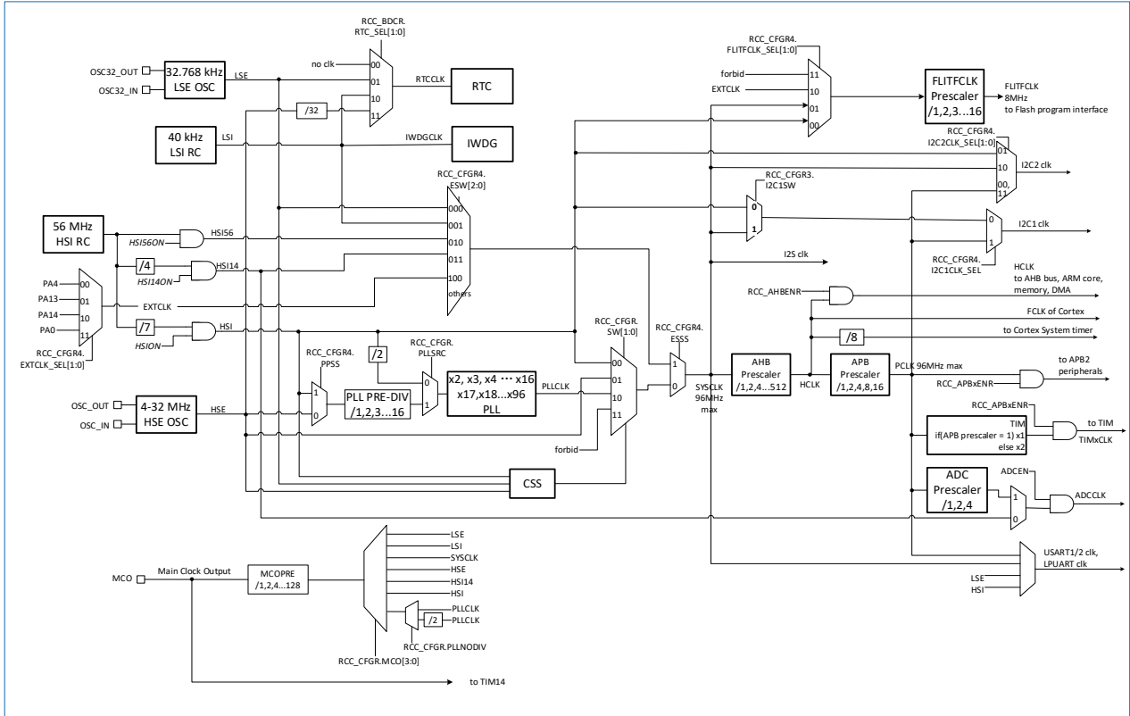
图 3-4 HK32F04AxxxxA 时钟树
