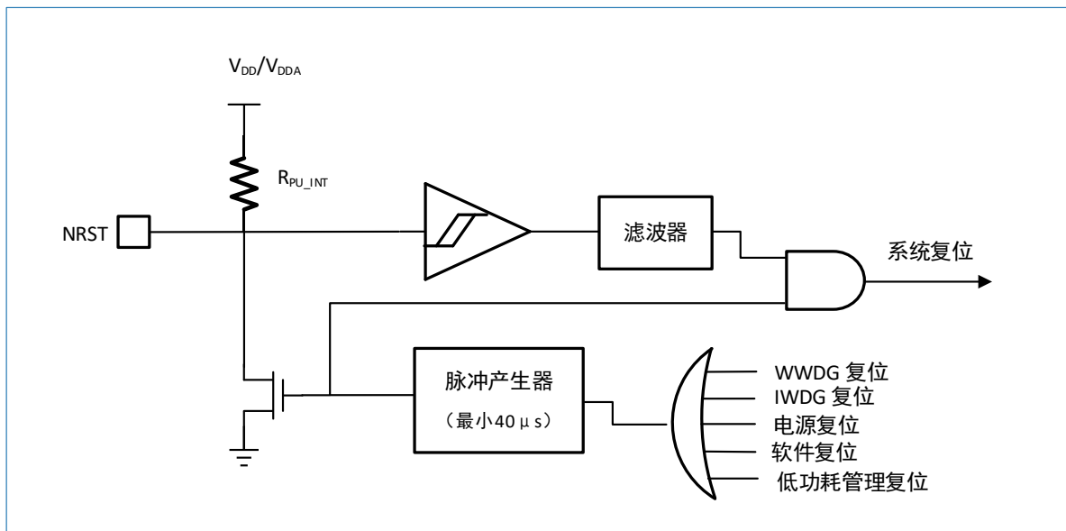
图 3-3 复位信号
