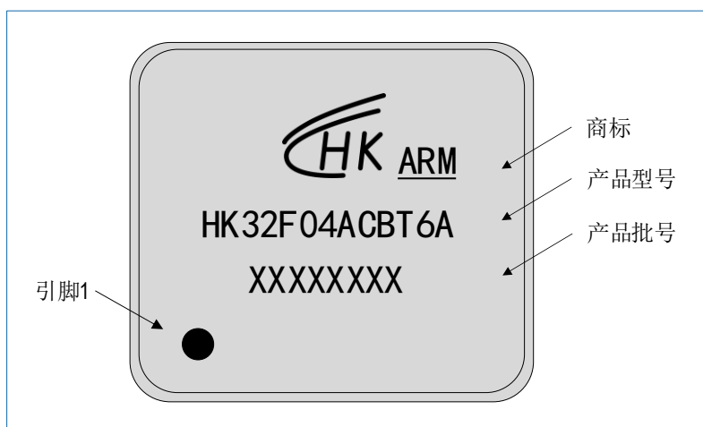
图 7-9 LQFP48 HK32F04ACBT6A 丝印示例
