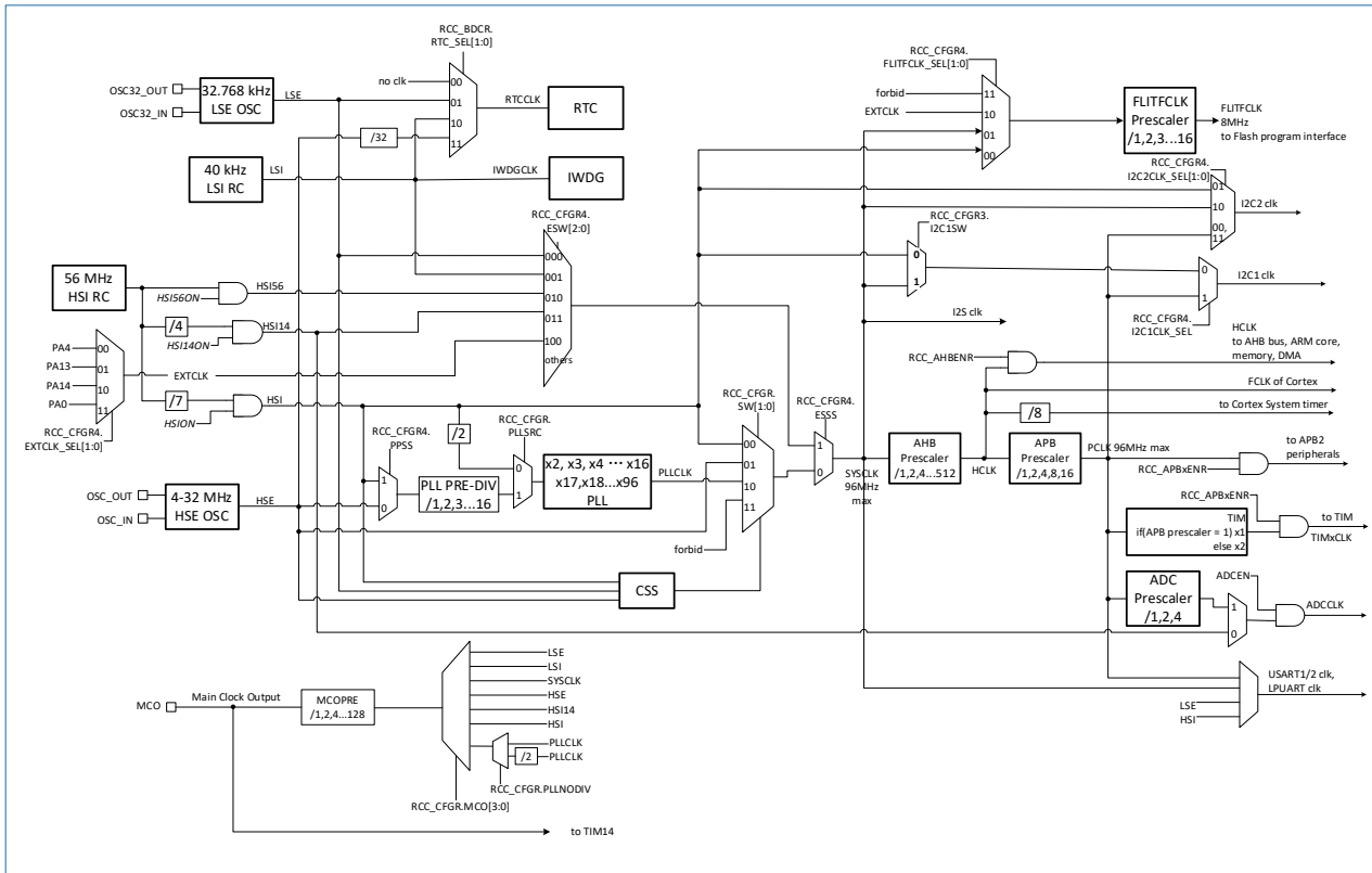
图 3-4 HK32F04AxxxxA 时钟树
