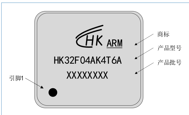
图 7-16 LQFP32 HK32F04AK4T6A 丝印示例
