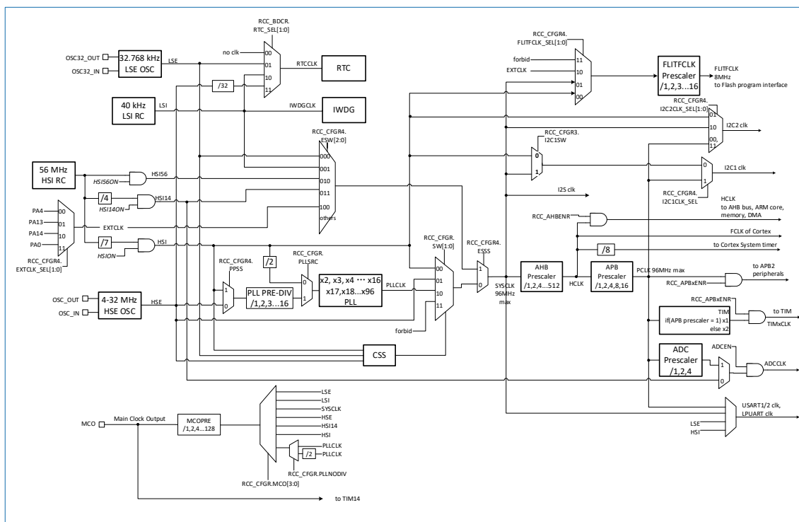
图 3-4 HK32F030xxxxA 时钟树
