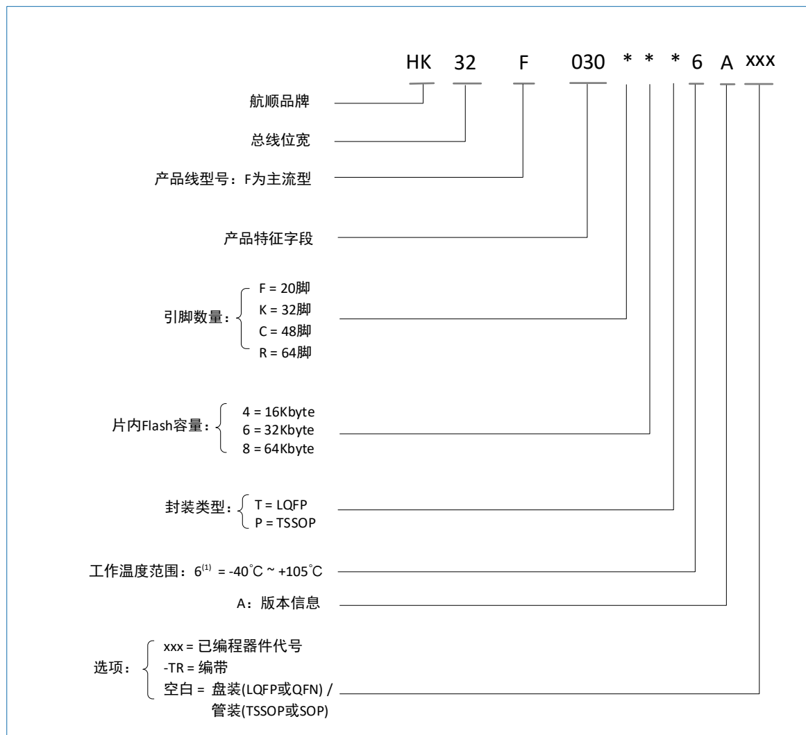
图 8-1 订货代码
