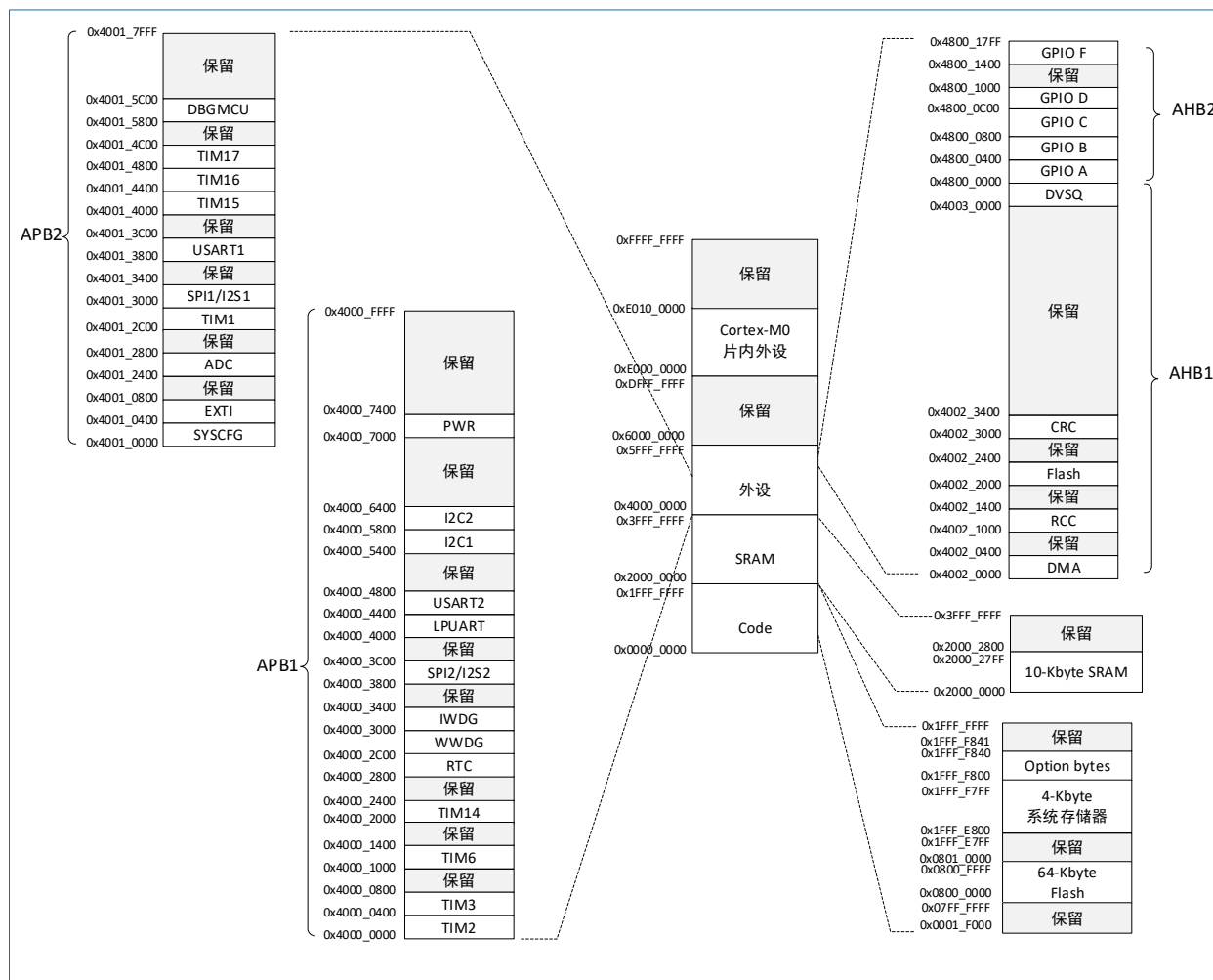
图 3-2 HK32F030R8T6A 存储器映射
