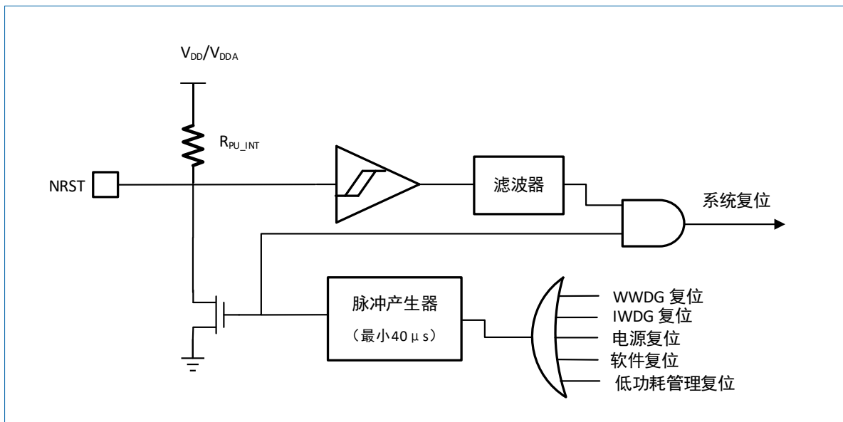
图 3-3 复位信号
