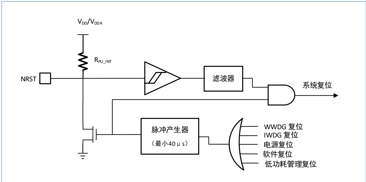
图 3-3 复位信号
