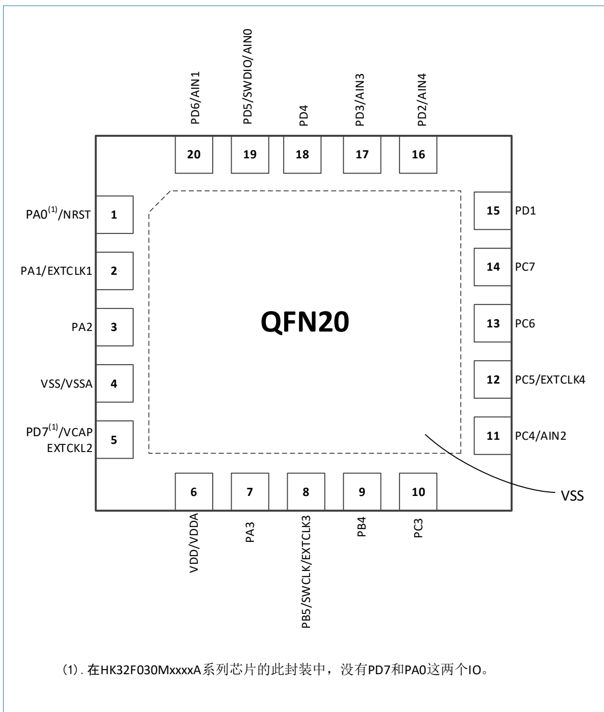
图 6-6 QFN20 封装引脚排列
