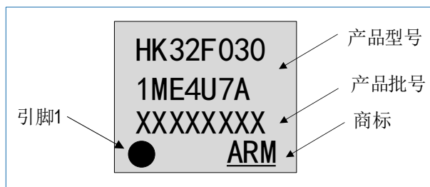
图 7-40 QFN24 HK32F0301ME4U7A 丝印示例
