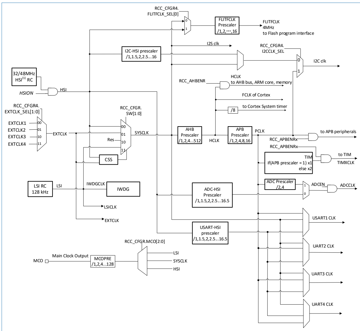
图 3-4 HK32F030MxxxxA/HK32F0301MxxxxA 时钟树
