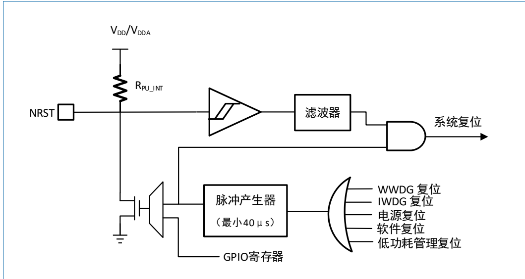
图 3-3 复位信号
