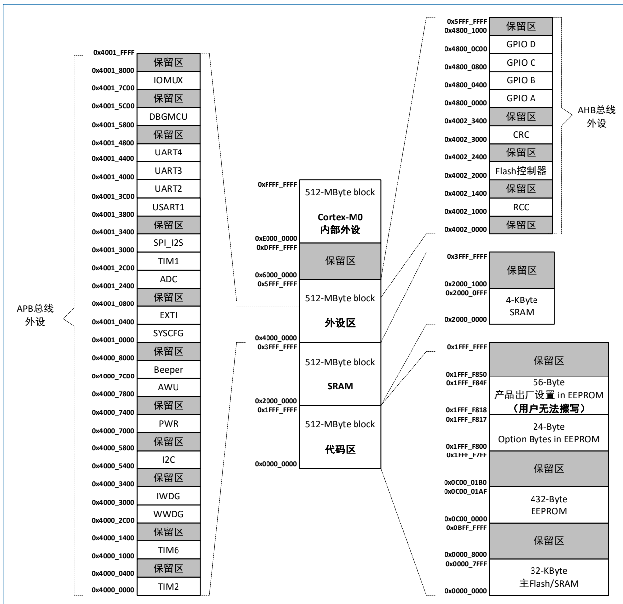
图 3-2 HK32F030MxxxA/HK32F0301MxxxA 存储器映射
