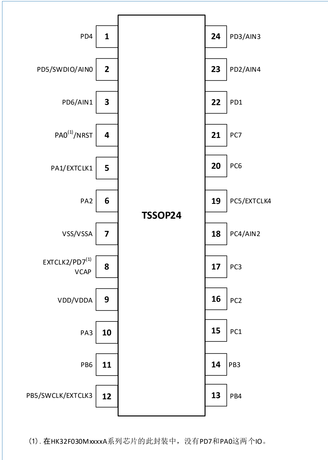
图 6-4 TSSOP24 封装引脚排列
