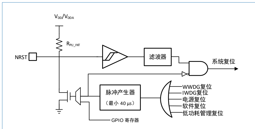
图 3-3 复位电路
