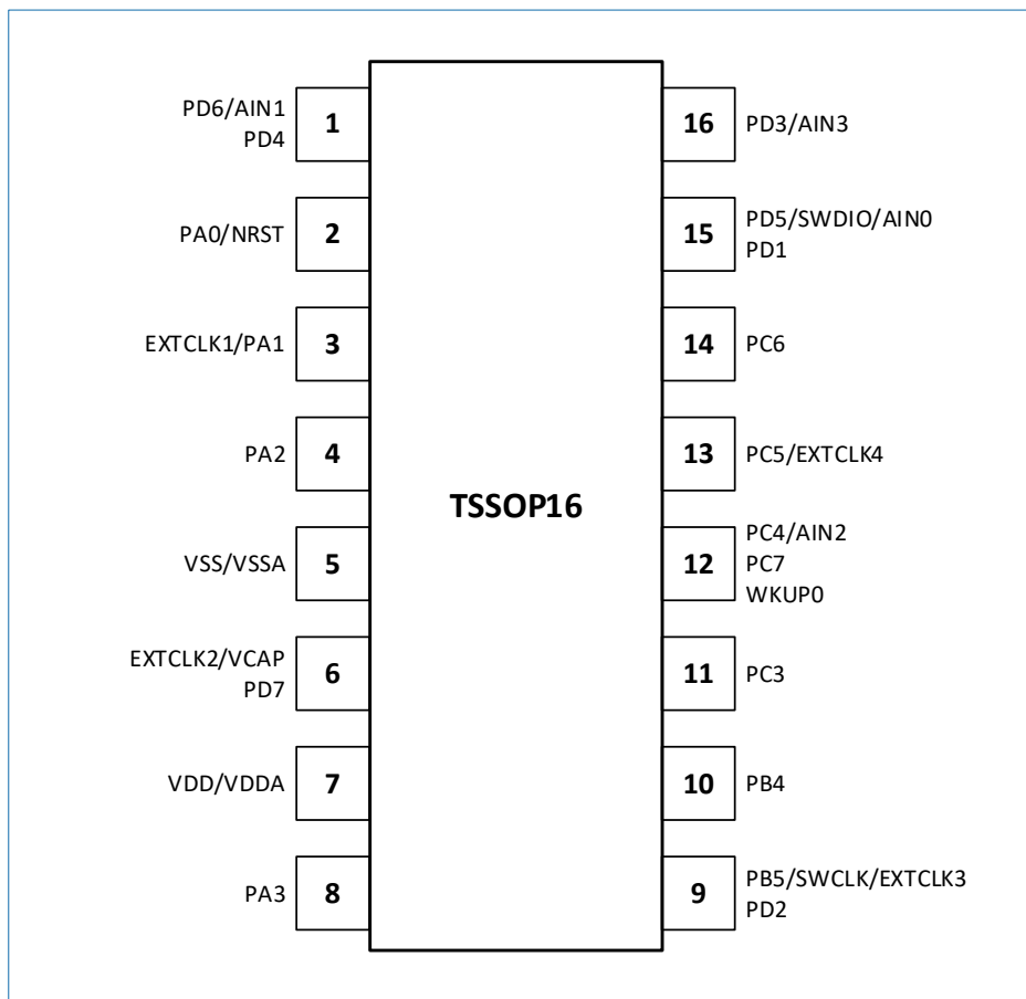
图 6-3 TSSOP16 封装
