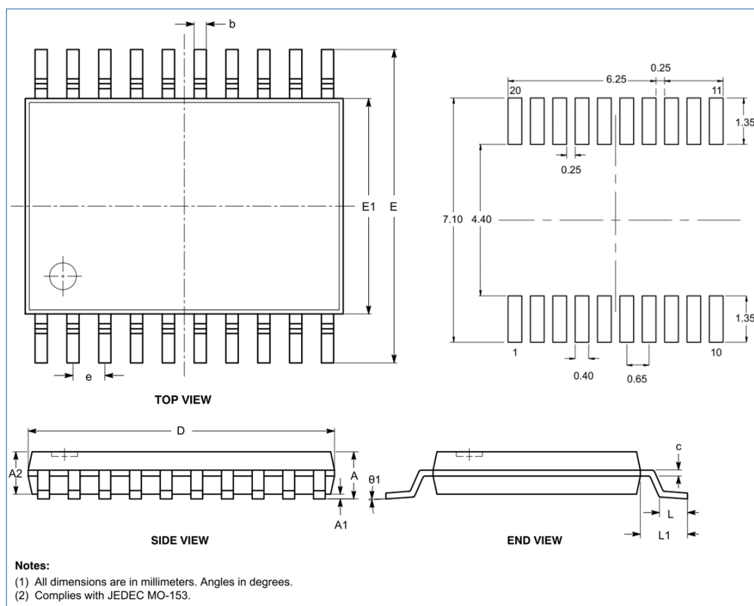
图 7-3 TSSOP20 封装尺寸图
