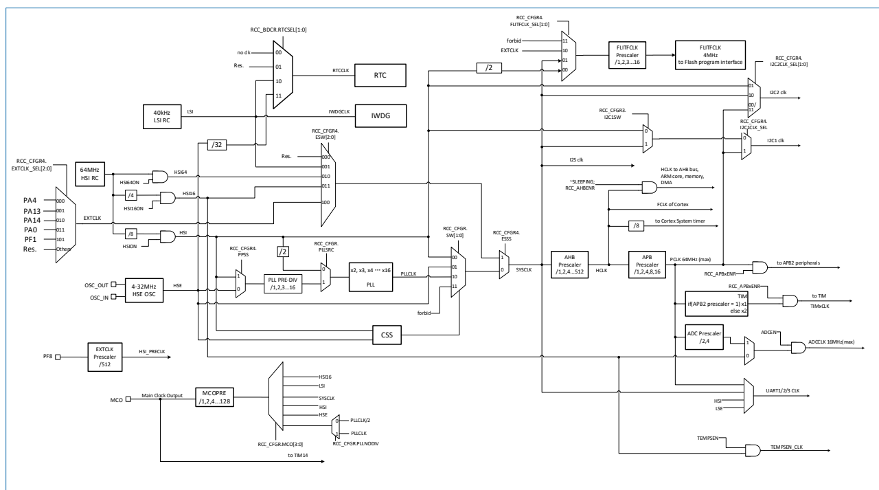
图 3-4 时钟树
