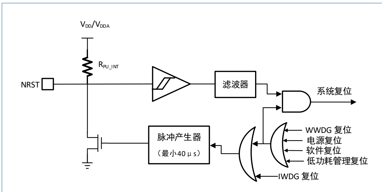
图 3-3 复位信号
