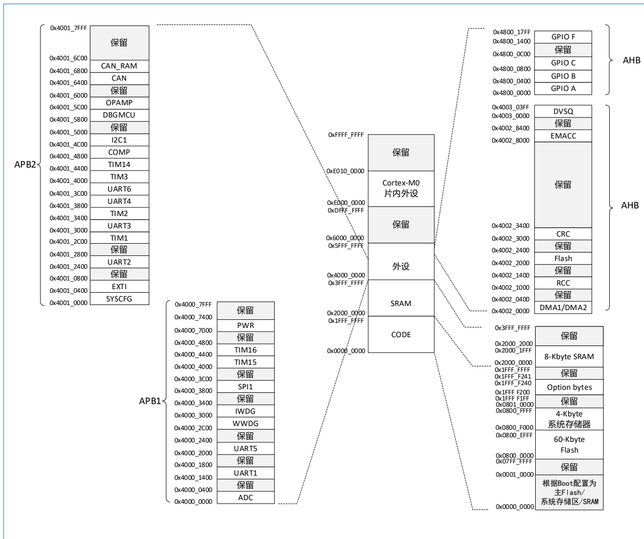
图 3-2 HK32ASPIN021C8T7 存储器映射
