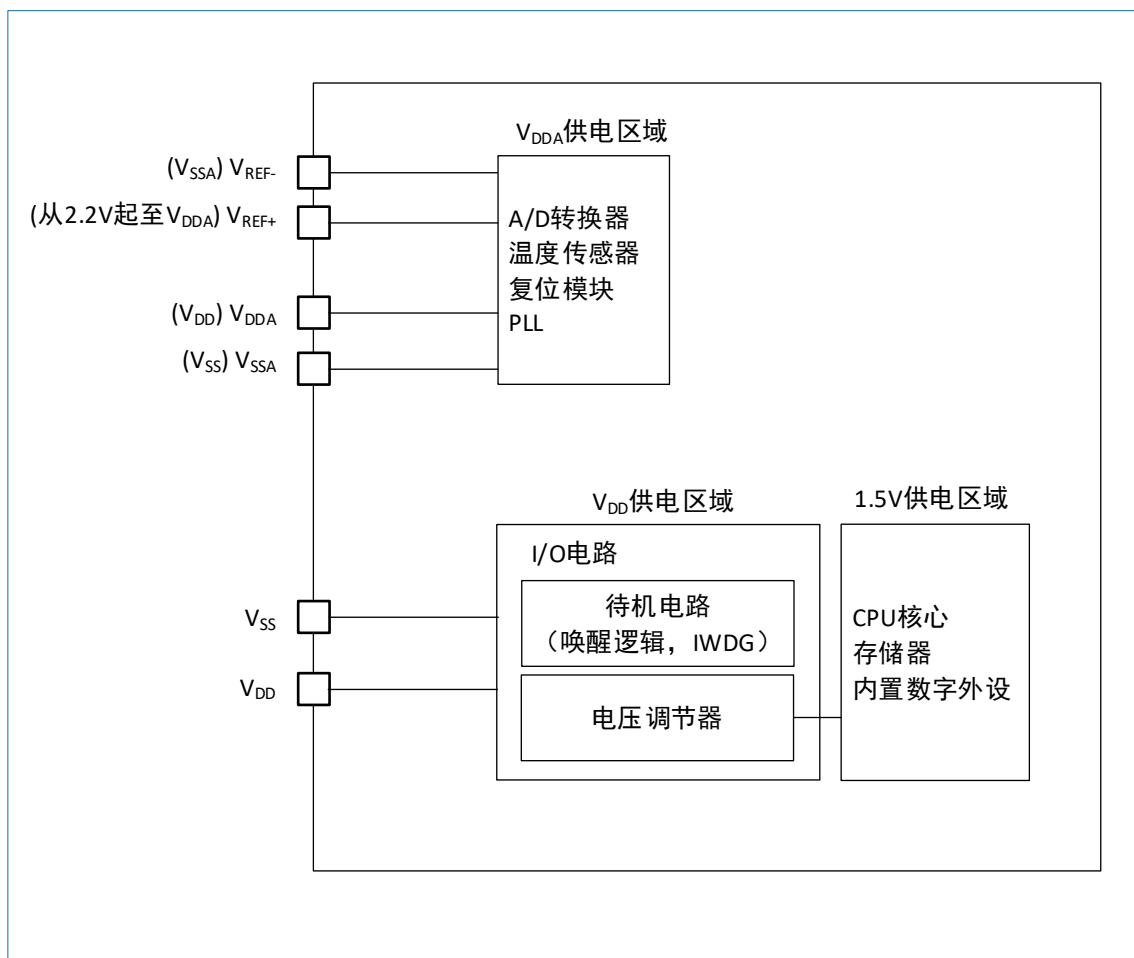
图 5-1 电源框图
