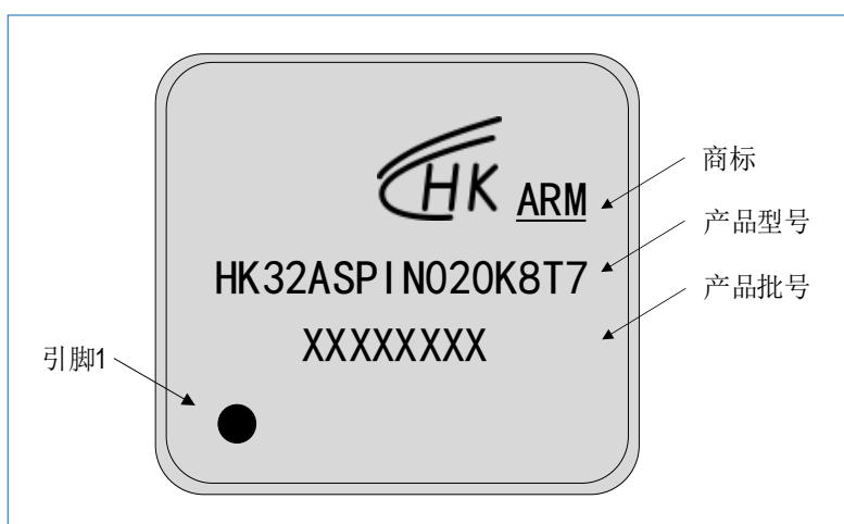
图 7-11 LQFP32 HK32ASPIN020K8T7 丝印示例
