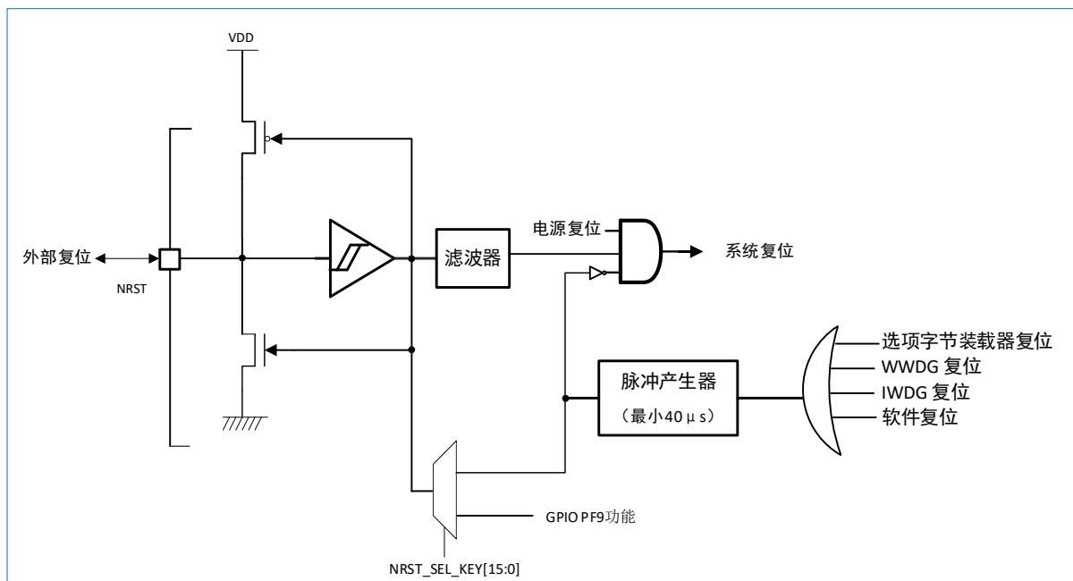
图 3-3 复位信号
