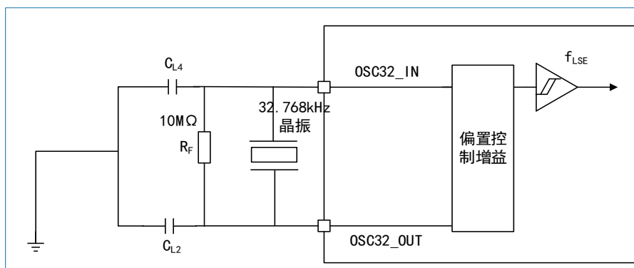
图 4-2 LSE 负反馈晶体振荡电路
