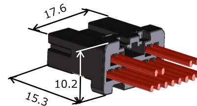
<Plug> ZE05-12DS-HU/R
