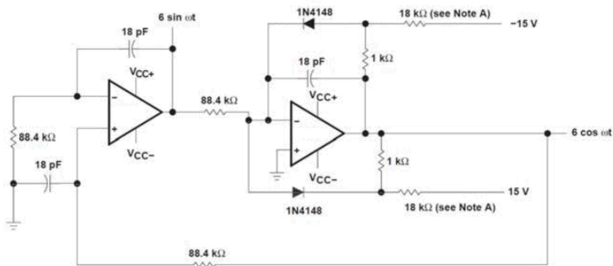
图 3. 100KHz 振荡器
