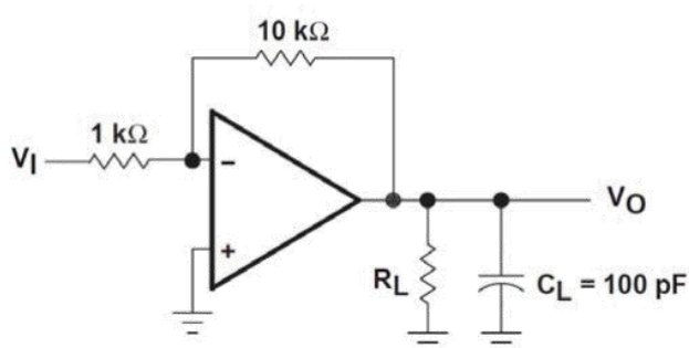
图 2. 10 倍增益电路
