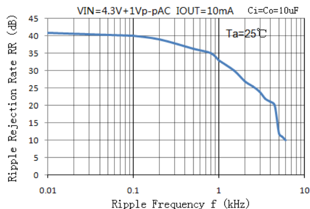
5、纹波抑制
