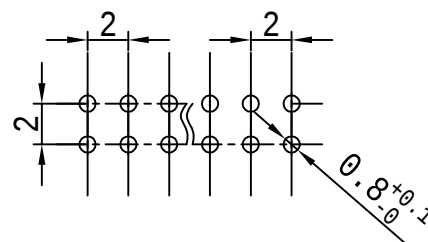
印制板开孔尺寸 ( \pm 0.1 )
