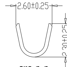
SEC:B-B
